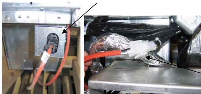
Figuur 3: Bevestig de twee-pins connectors wit en sluit de zwarte connector in het nut doos zoals afgebeeld.
